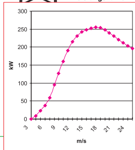
Leistungskurve
